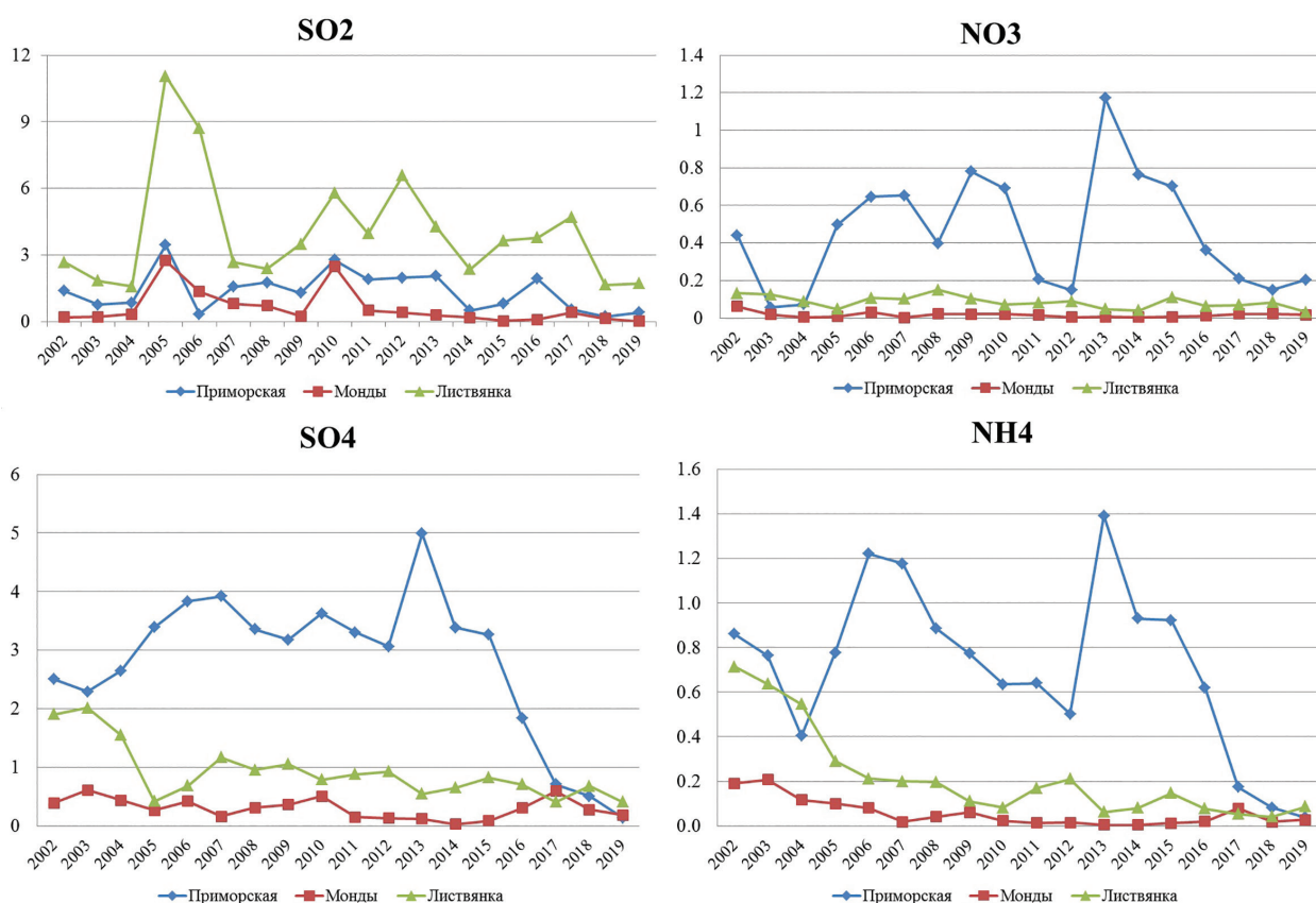
Рисунок 2.12 – Изменения средних годовых концентрации соединений серы (сверху) и азота (снизу) в воздухе на станциях ЕАНЕТ (мкг/м 3 )
