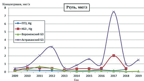
Рисунок 2.8 – Динамика среднего содержания ртути в атмосферных осадках фоновых районов, 2009-2019 гг.
