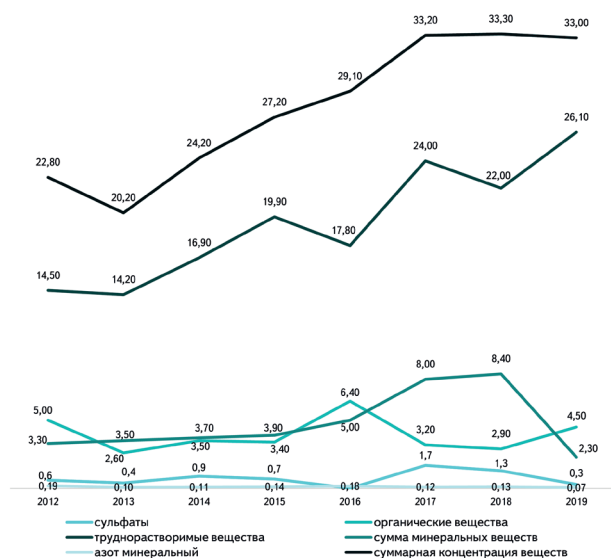
Рисунок 12.5 – Динамика поступления химических веществ из атмосферы на ст. Хужир, тонн/год на км 2
