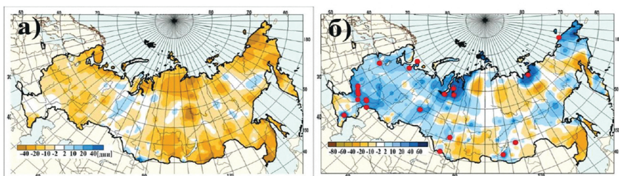
Рисунок 3.10 – а) аномалии числа дней с покрытием снегом более 50 % территории вокруг метеостанции зимой 2018-2019 гг. (от среднеемноголетних значений за период 1971-2000 гг.); б) аномалии максимальной высоты снежного покрова зимой 2018-2019 гг. (от средних многолетних значений за период 1971-2000 гг.). Точками красного цвета показаны станции, на которых зарегистрирован абсолютный максимум высоты снежного покрова.
