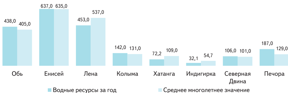
Рисунок 11.12 – Ресурсы речного стока в речных бассейнах в сравнении со средним многолетним значением, км 3
