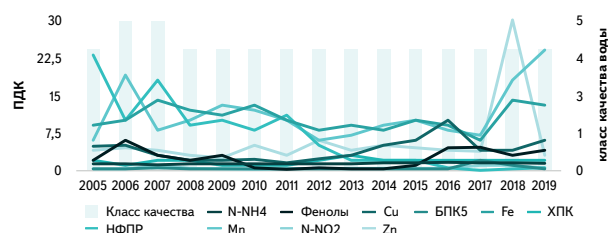
Рисунок 4.17 – Динамика среднегодовых концентраций отдельных загрязняющих веществ и качества воды р. Обь ниже г. Салехард, 2005-2019 гг.
