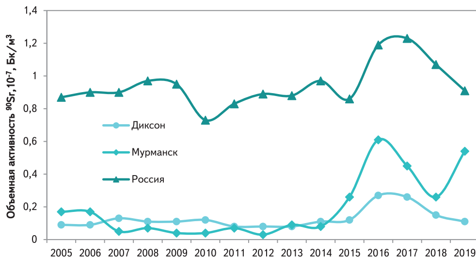
Рисунок 11.28 – Динамика объемной активности 90 Sr в воздухе на о. Диксоне, в Мурманске и средневзвешенной по Российской Федерации в 2005-2019 гг.
