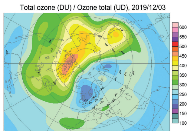
Рисунок 3.21 – Поле значений ОСО (ед. Д.) 3 декабря 2019 г. по данным Мирового центра данных ВМО по озону и ультрафиолетовой радиации
