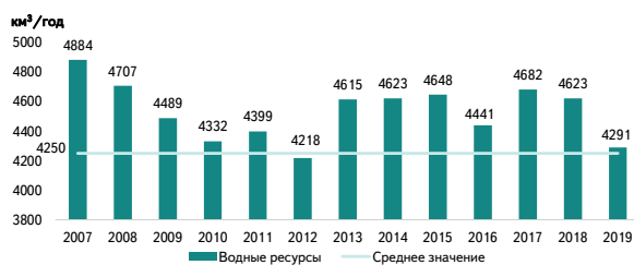
Рисунок 4.3 – Динамика водного стока в Российской Федерации, 2007-2019 гг., км 3
