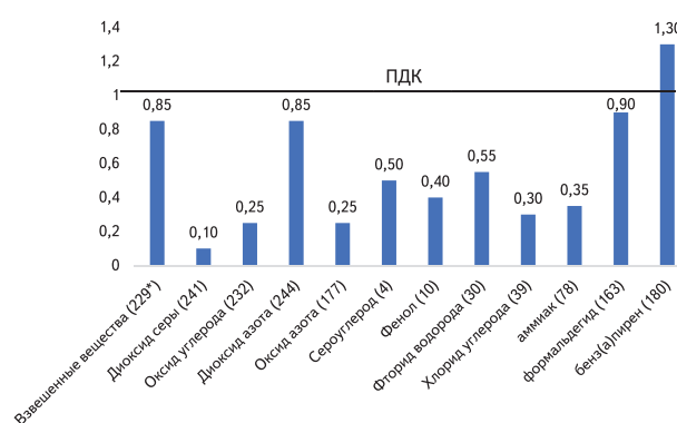
Рисунок 2.24 – Средние за год концентрации примесей относительно ПДК в городах Российской Федерации, q ср /ПДК
