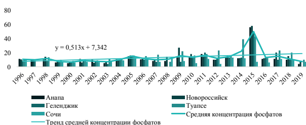
Рисунок 4.36 – Динамика средней концентрации фосфатов P-PO_4 (мг/дм 3 ) в прибрежных водах Кавказа, 1996-2019 гг.
