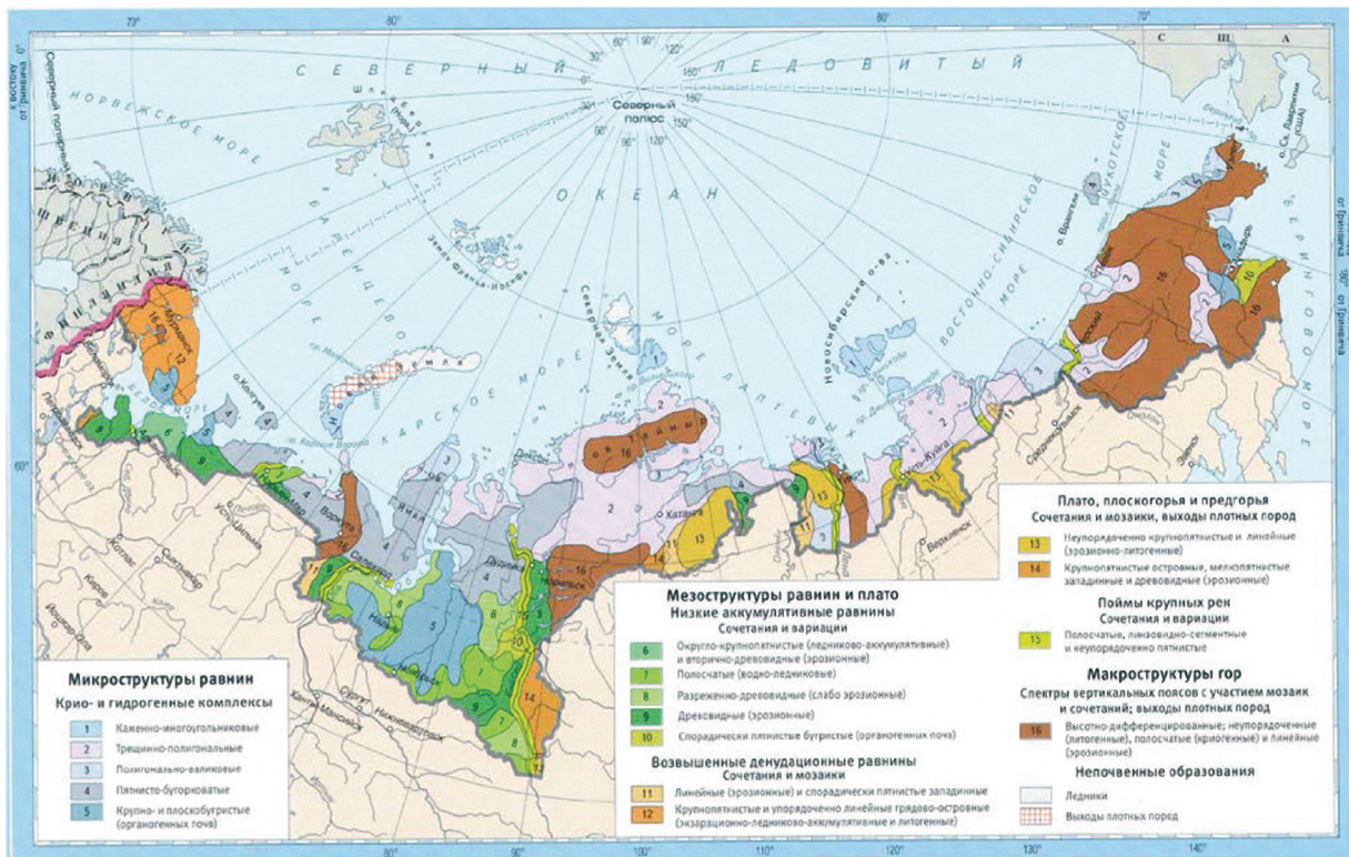
Рисунок 11.15 – Структура почвенного покрова Арктической зоны Российской Федерации
