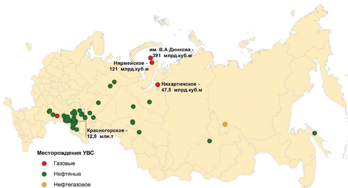
Рисунок 5.2 – Месторождения углеводородного сырья, открытые в 2019 г.
