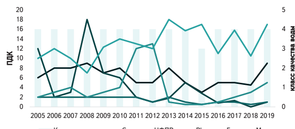
Рисунок 4.21 – Динамика среднегодовых концентраций отдельных ингредиентов и качества воды р. Колыма, п. Усть-Среднекан, 2005-2019 гг.
