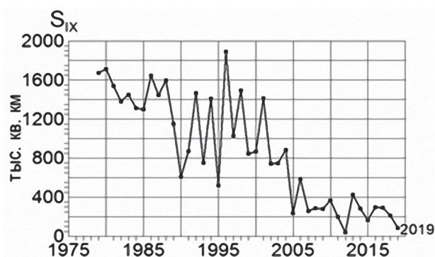
Рисунок 11.10 – Площадь, занятая морским льдом в сентябре в Сибирских арктических морях (моря Карское, Лаптевых, Восточно-Сибирское, Чукотское) по данным отдела ледовых прогнозов ААНИИ
