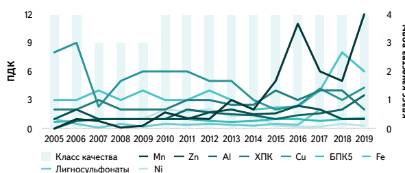
Рисунок 4.6 – Динамика среднегодовых концентраций отдельных ингредиентов и качества воды р. Северная Двина, г. Красавино, 3,5 км ниже города, 2005-2019 гг.
