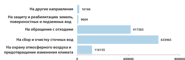
Рисунок 14.5.33 – Текущие (эксплуатационные) затраты на охрану окружающей среды, тыс. руб.
