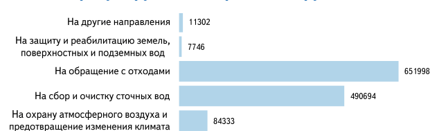
Рисунок 14.1.17 – Текущие (эксплуатационные) затраты на охрану окружающей среды, тыс. руб.
