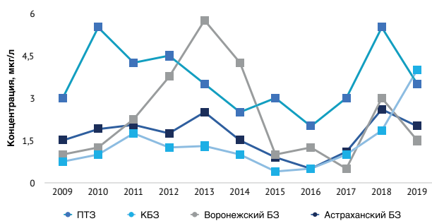
Рисунок 2.6 – Динамика среднего содержания свинца в атмосферных осадках фоновых районов, 2009-2019 гг.
