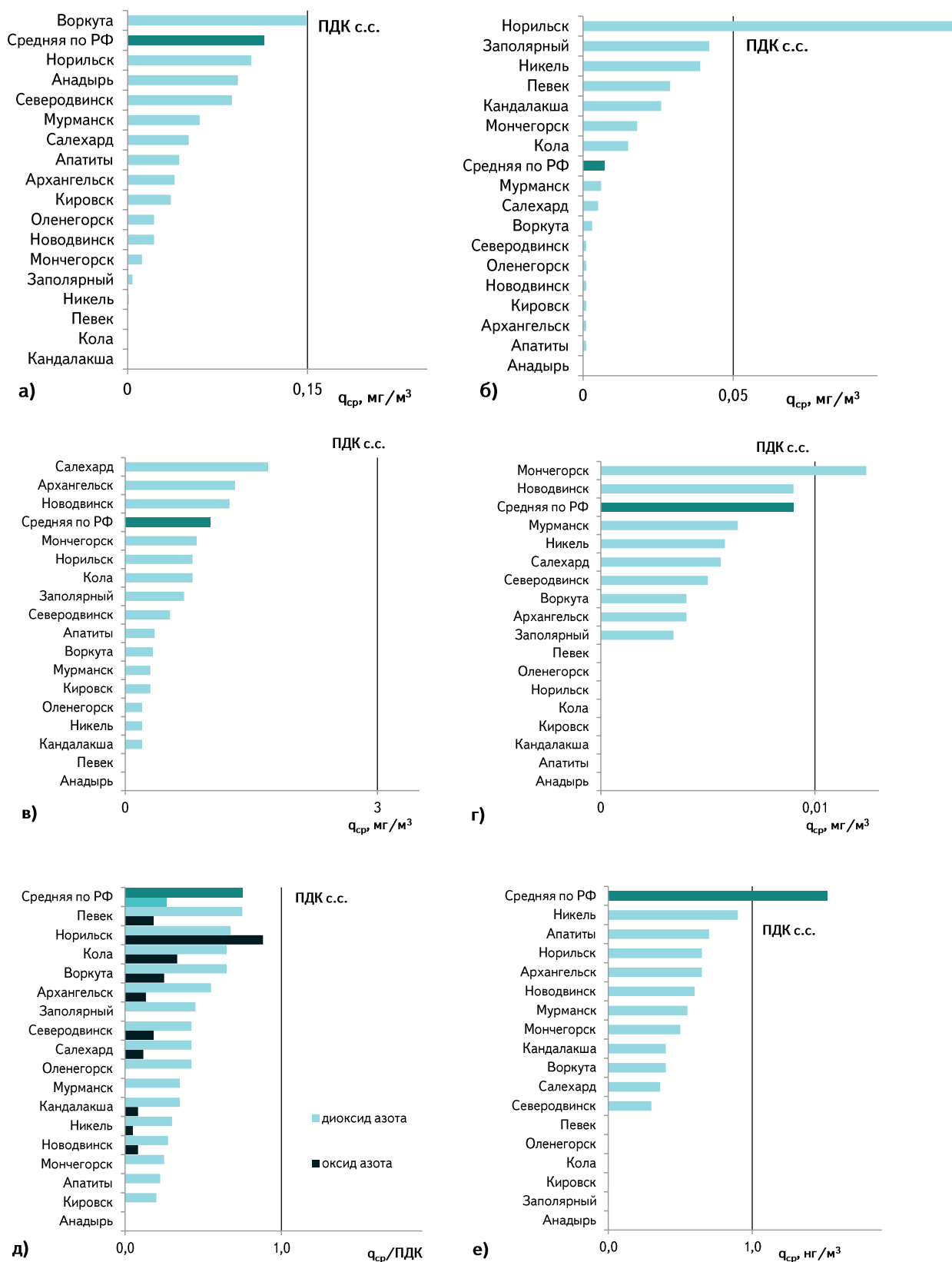
Рисунок 11.30 – Средние за год концентрации: взвешенных веществ (а), диоксида серы (б), оксида углерода (в), формальдегида (г), q_{ср} , мг/м 3 , диоксида и оксида азота (д), q_{ср} , ПДК, бенз(а)пирена (е), q_{ср} , нг/м 3 , в городах Арктической зоны Российской Федерации и в целом по Российской Федерации в 2019 г.
