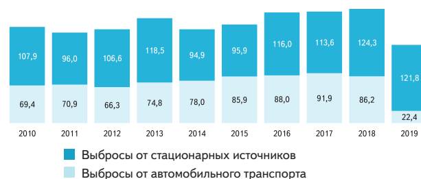
Рисунок 14.2.18 – Динамика выбросов загрязняющих веществ в атмосферный воздух в 2010–2019 гг., тыс. т
