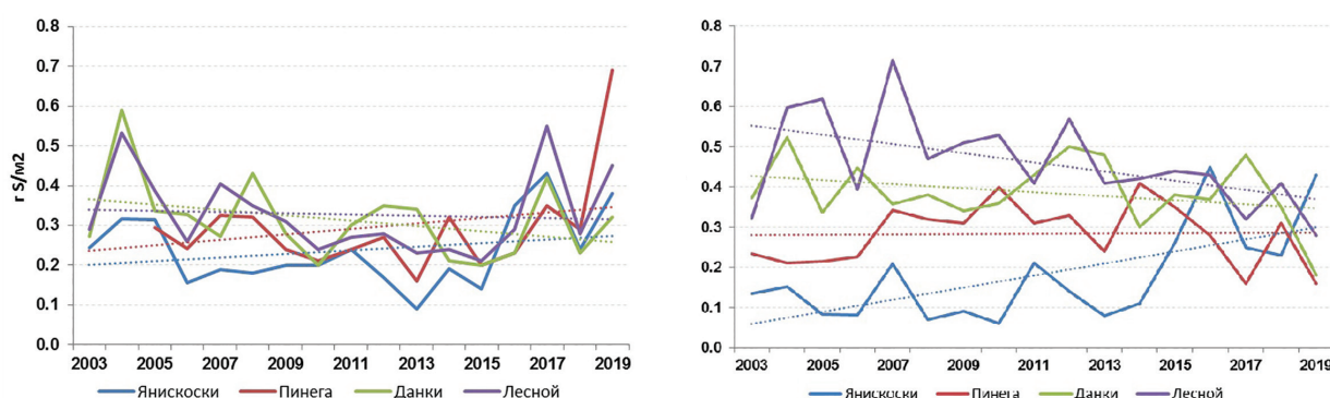
Рисунок 2.10 – Многолетние выпадения сульфатной серы (слева) и суммарного нитратного и аммонийного азота (справа) из атмосферы с осадками на станциях ЕМЕП (г N/м 2 в год)
