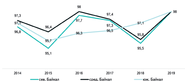
Рисунок 12.6 – Минерализация воды озера по котловинам продольного разреза, мг/л
