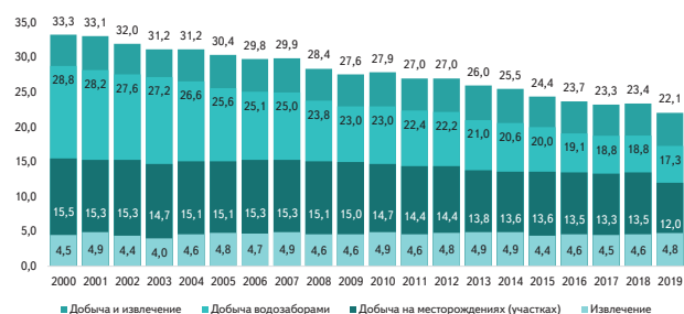
Рисунок 4.62 – Динамика изменения добычи и извлечения питьевых и технических подземных вод по территории Российской Федерации, млн м 3 /сут
